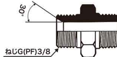
【1013管用アダプター(おすシート)タイプ】
