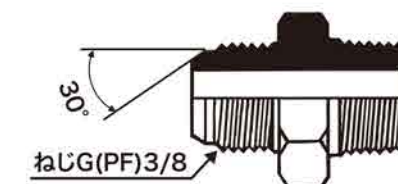
【1013管用アダプター(おすシート)タイプ】
