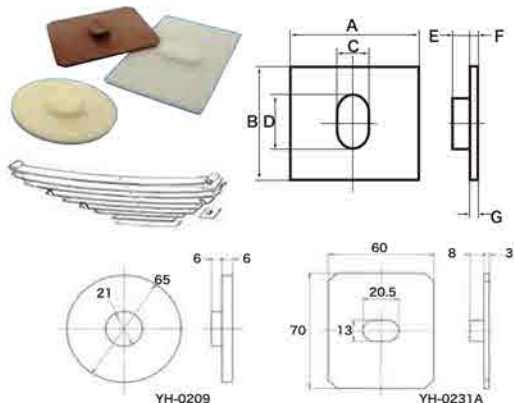
リーフスプリングパッドサイズ表 (mm)
