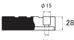
穴径断面図
